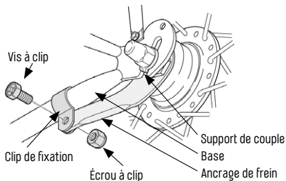
Fig. 3/21 Ancrage à frein Source Shimano
