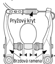
Obr. 3/18 Zdroj Shimano
