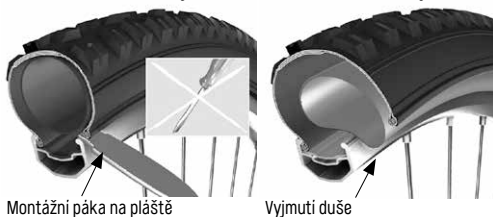
Obr. 4/34 Zdroj Schwalbe
