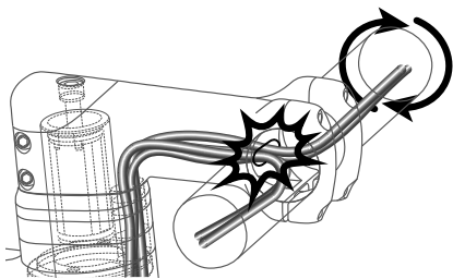
Obr. 1/16 Uvnitř uložená brzdová vedení a lanovody řazení
