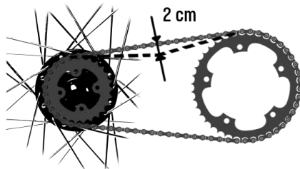
Obr. 4/21 Napětí řetězu
