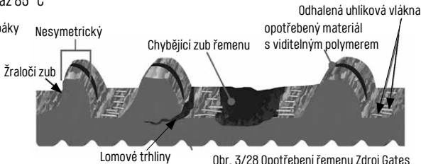
Obr. 3/28 Opotřebení řemenu Zdroj Gates
