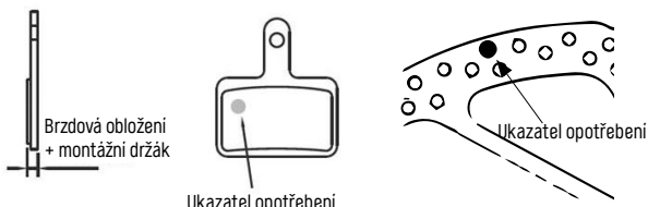
Obr. 1/21 Zdroj Tektro
