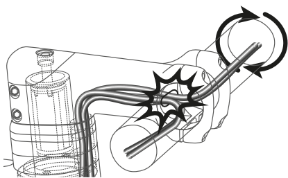
Obr. 1/24 Vnútorne vedené brzdové lanká a lanká radenia
