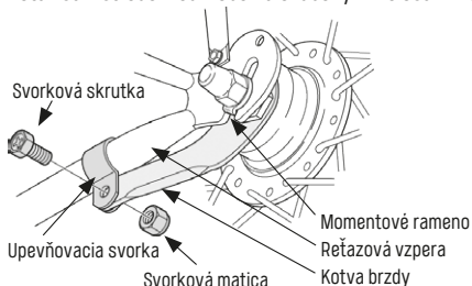
Obr. 3/29 kotva brzdy, zdroj Shimano
