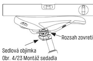
Obr. 4/23 Montáž sedadla
