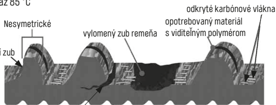
Obr. 3/36 opotrebovanie remeňa, zdroj Gates
