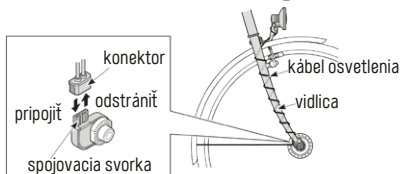
Obr. 2/49 Spojovacia svorka nábojového dynamo zdroj: Shimano
